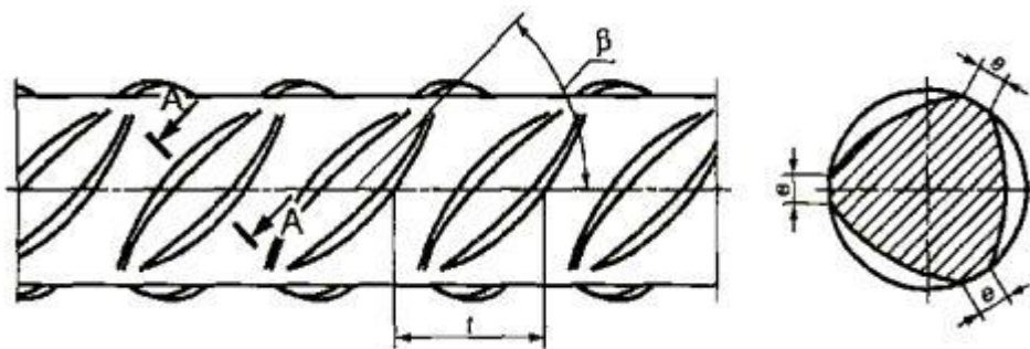
Рисунок А.2 - Трехсторонний серповидный периодический профиль холоднореформированного арматурного проката
