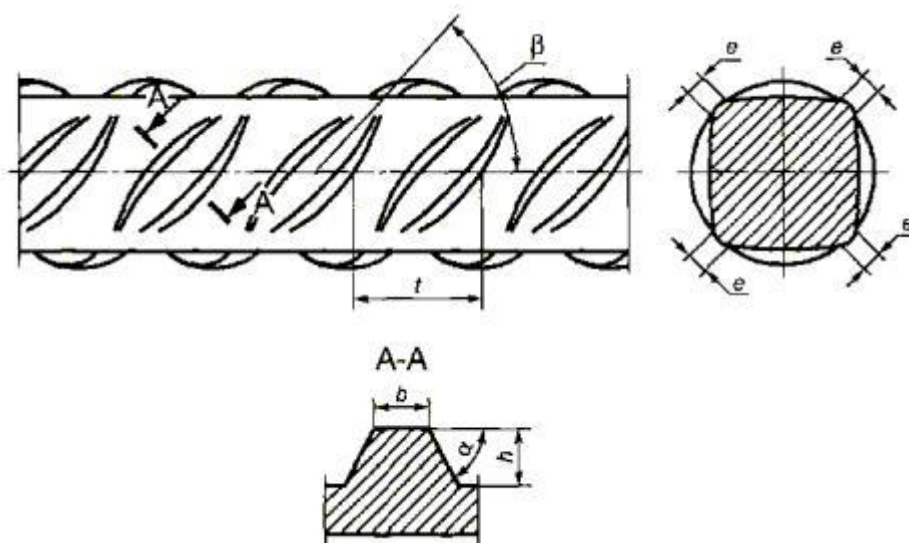
Рисунок А.3 - Четырехсторонний сегментный периодический профиль холоднореформированного арматурного проката
