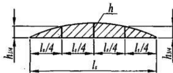
Рисунок 2 - Поперечное сечение ребра (сечение А-А из рисунка 1)
